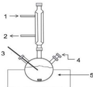
Hình 1: Sơ đồ thí nghiệm điều chế methyl acrylate từ acid và alcohol tương ứng.
